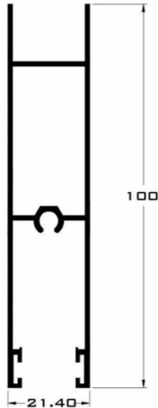
3560 ZOCALO
