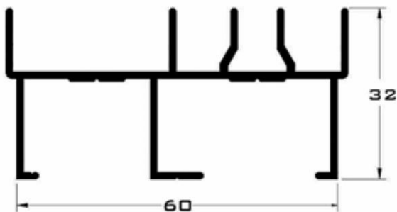
3508 CERCO LATERAL
