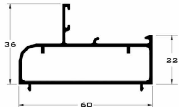
3510 FIJO TUBULAR
