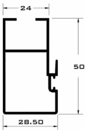
3504 HOJA CENTRAL
