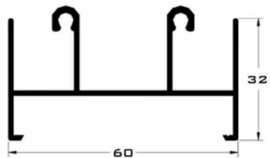
3502 CERCO SUPERIOR
