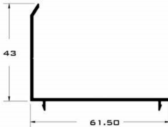
3512 SOLAPE EMBELLECEDOR
