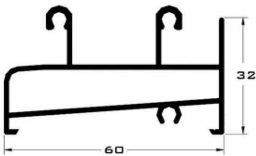
3501 CERCO INFERIOR
