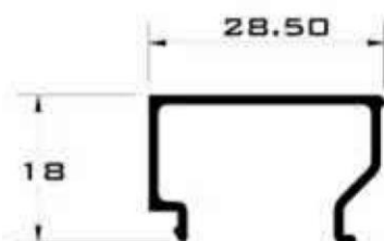
1430 JUNQUILLO ANCHO
