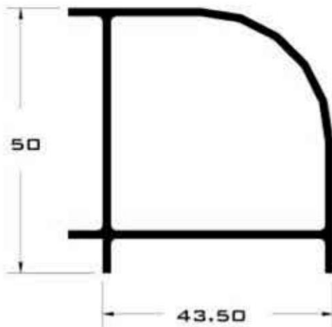
1427 ESQUINERO REDONDO
