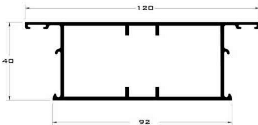
1423 HOJA MONUMENTAL
