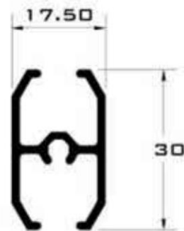
2516 CUADRICULA
