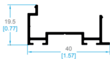
61446 ARRASTRE PUERTA
