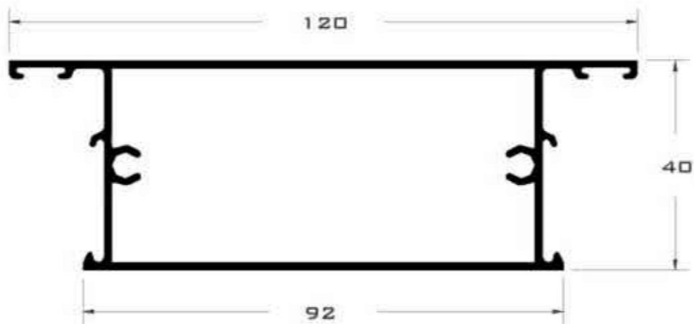
1422 ZOCALO CENTRAL
