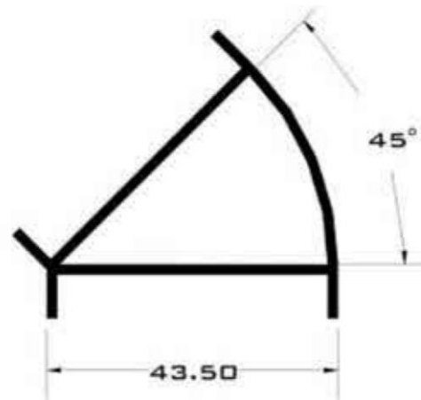
1428 ESQUINERO REDONDO 45°
