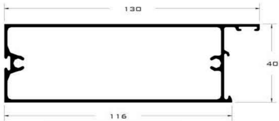
1434 ZOCALO INFERIOR
