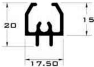
2415 RECERCADO
