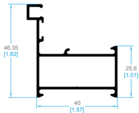
61448 JUNQUILLO 24 mm
