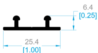
3316 RIEL VITRINA.
