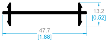
7792 MOLDURA UNIÓN.
