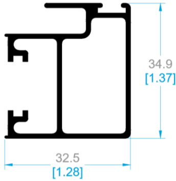
7844 TRASLAPE VENTANA.
