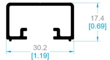
8681 CERCO FIJO.
