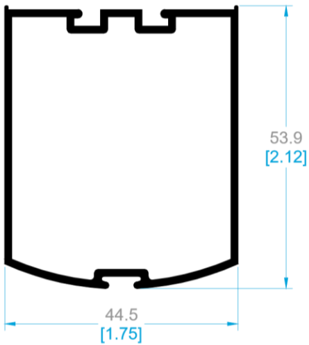
9204 CERCO CHAPA.
