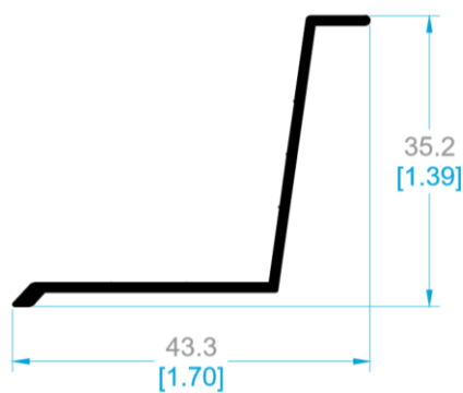
1439 PERIFL PARA DOMO.
