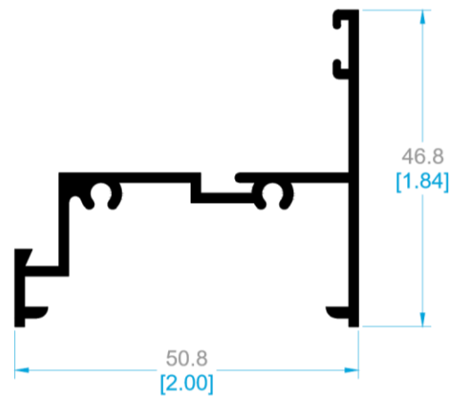
8937 CONTRAMARCO.
