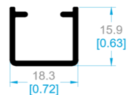
7525 CERCO FIJO ECONÓMICO.
