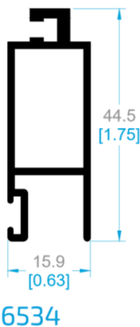
MOSQUITERO VERTICAL.
