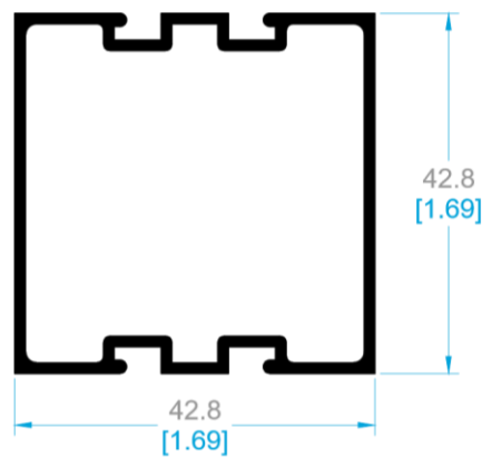
9183 INTERMEDIO.
