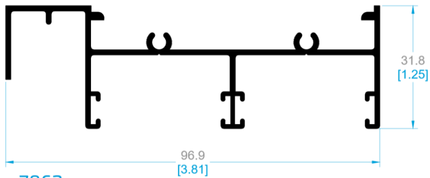
7862 CHAMBRANA CON MOSQUITERO.
