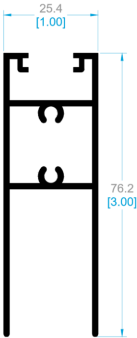
7842 ZOCLO PUERTA.
