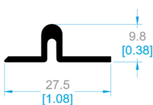
7818 RIEL ADAPTADOR.
