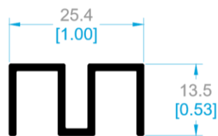
3329 GUÍA VITRINA.
