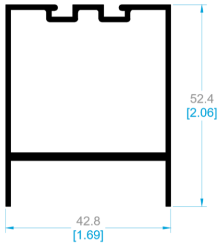
9207 CABEZAL.
