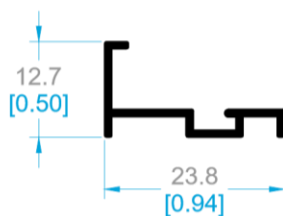
7013 PORTAVIDRIO.
