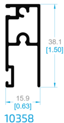
MOSQUITERO UNIVERSAL.
