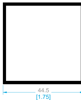
11093 TUBO CUADRADO DE 1\frac{3}{4} ".
