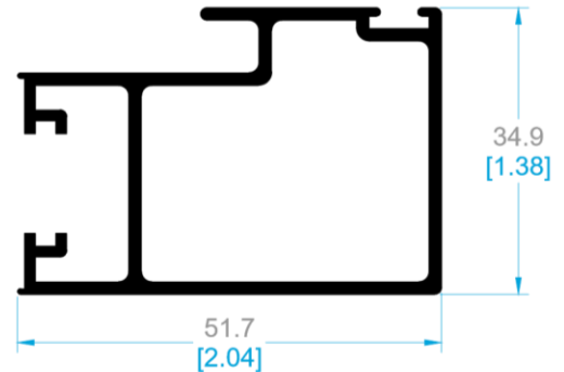
7848 TRASLAPE PUERTA.
