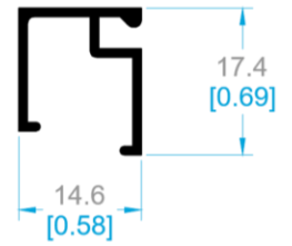
6370 JUNQUILLO.
