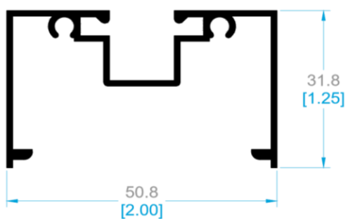
9083 BOLSA.
