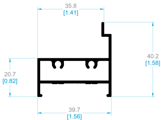
2230 CONTRAMARCO.
