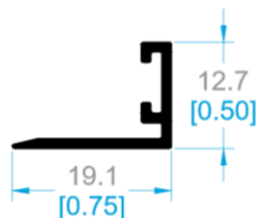
11032 BATIENTE.
