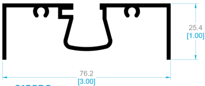
9135BC BOLSA CORTA.
