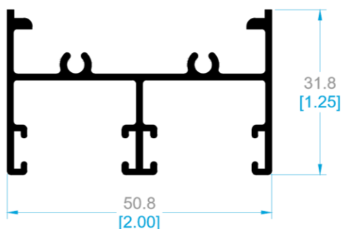
7518 CHAMBRANA.
