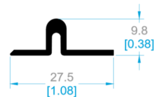
RIEL ADAPTADOR.
