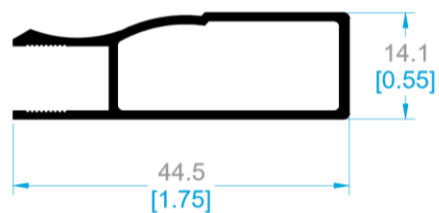
9756 MARCO SEMILUJO.
