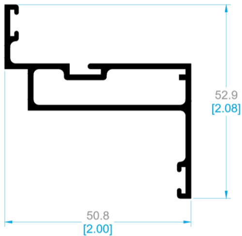
8936 MARCO.
