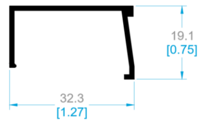
9112 JUNQUILLO.
