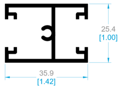
9082 INTERMEDIO.
