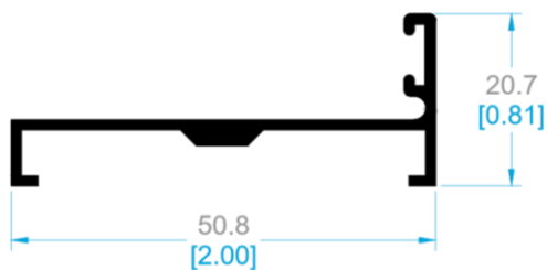
5844 BATIENTE.
