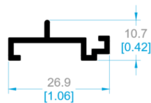
ADAPTADOR MOSQUITERO.
