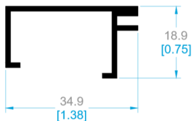
8939 JUNQUILLO.
