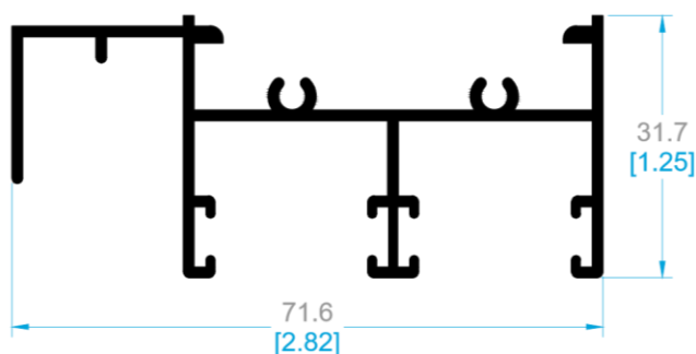
7819 CHAMBRANA CON MOSQUITERO.
