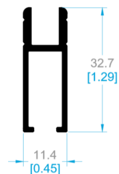
3358 ZAPATA VITRINA.
