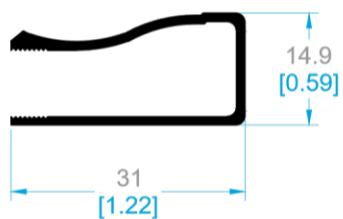
9525 MARCO ECONÓMICO.
