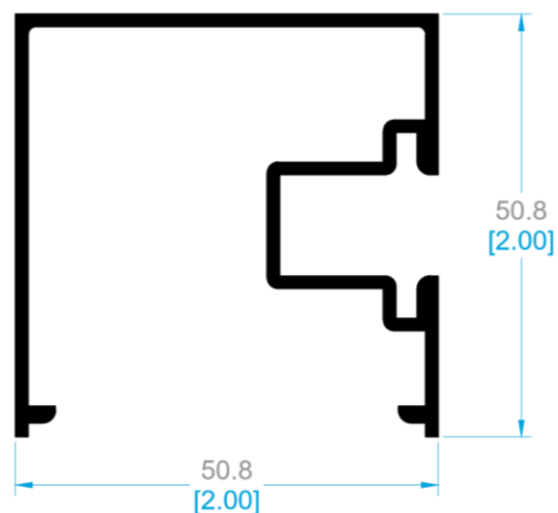
8586 ESQUINERO.
