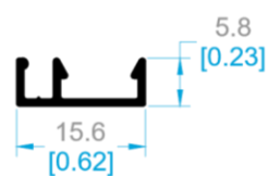
MOSQUITERO LIGERO.
