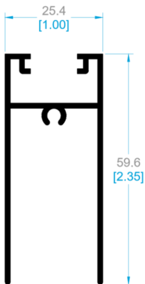
7835 ZOCLO VENTANA.
