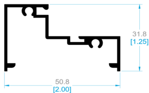
9084 ESCALONADO.
