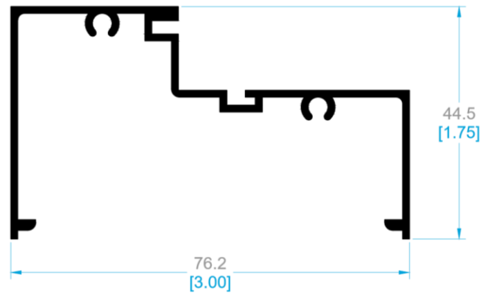
9136 ESCALONADO.
