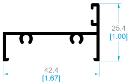
8550 BATIENTE CON VENAS.
