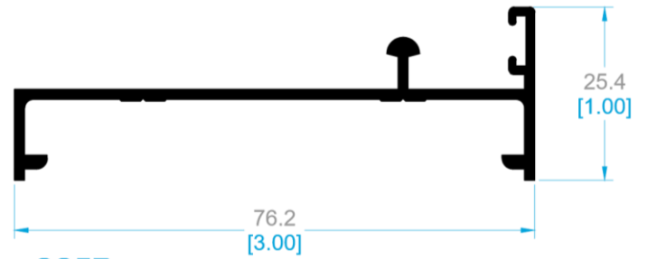
9957 RIEL.
