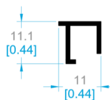
7014 JUNQUILLO.
