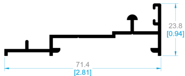
8370 RIEL CON MOSQUITERO.
