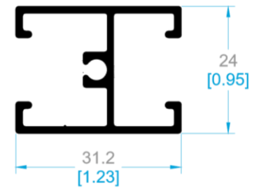
9081 INTERMEDIO CORTO.
