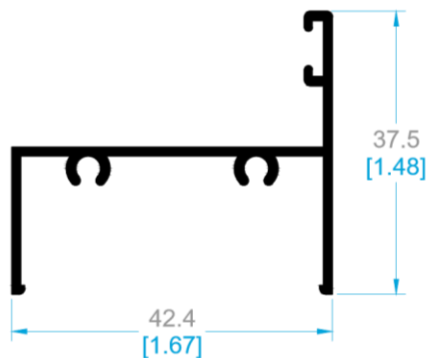
8570 BATIENTE.
