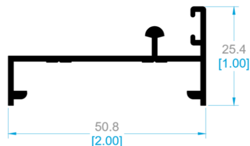
9953 RIEL.
