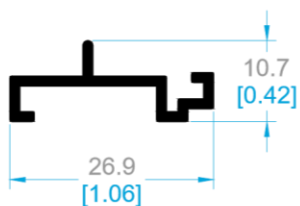
9966 ADAPTADOR MOSQUITERO.
