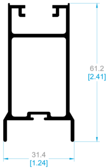
7850 CERCO OXXO.
