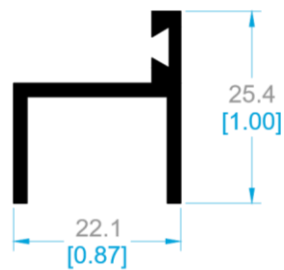
7102 BATIENTE.
