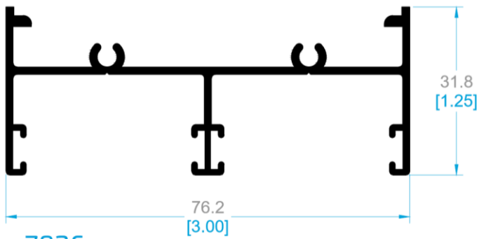
7826 CHAMBRANA.
