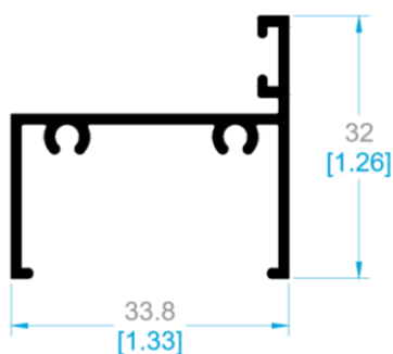
8560 BATIENTE LARGO.
