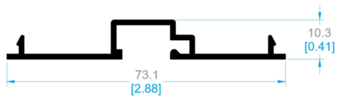
10237 TAPA BOLSA CORTA.
