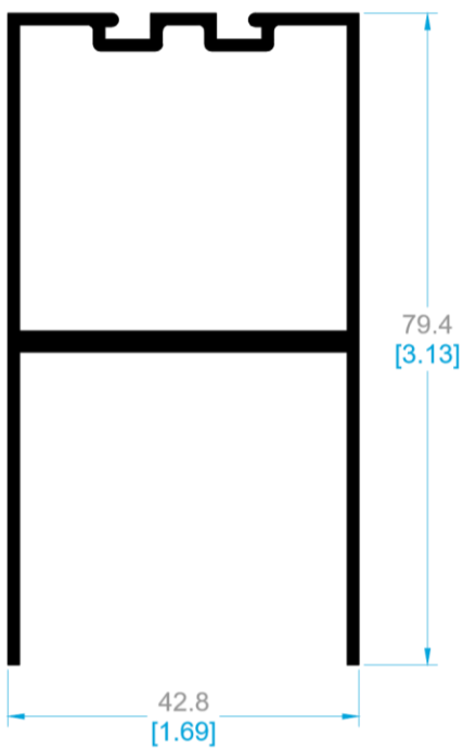
9187 ZOCLO.
